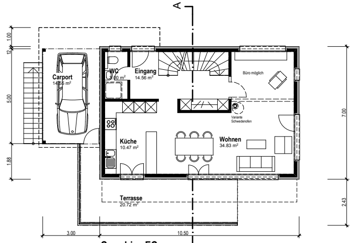
Grundriss EG
