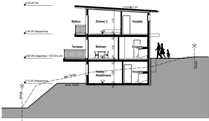
Schnitt A-A
