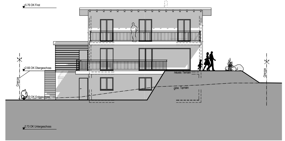
Süd-West Fassade
