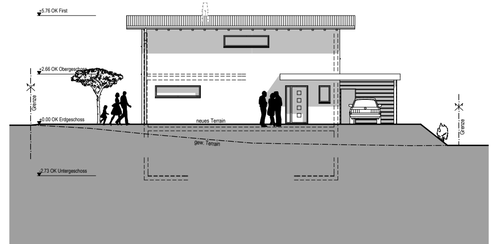
Nord-Ost Fassade
