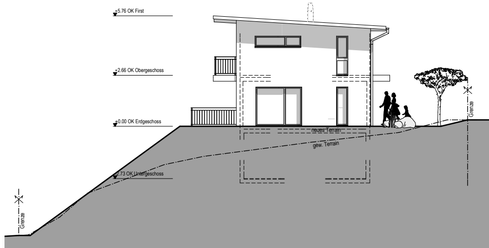
Süd-Ost Fassade
