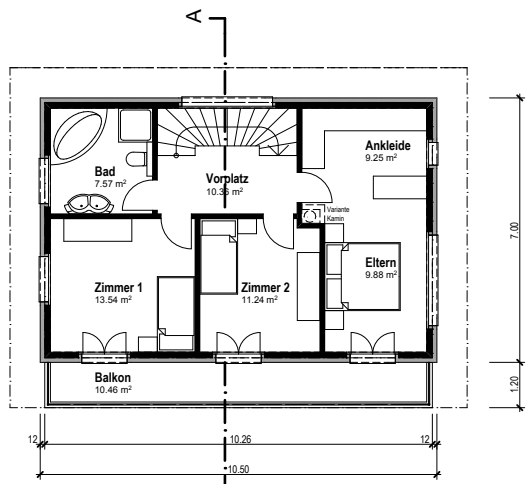
Grundriss DG
