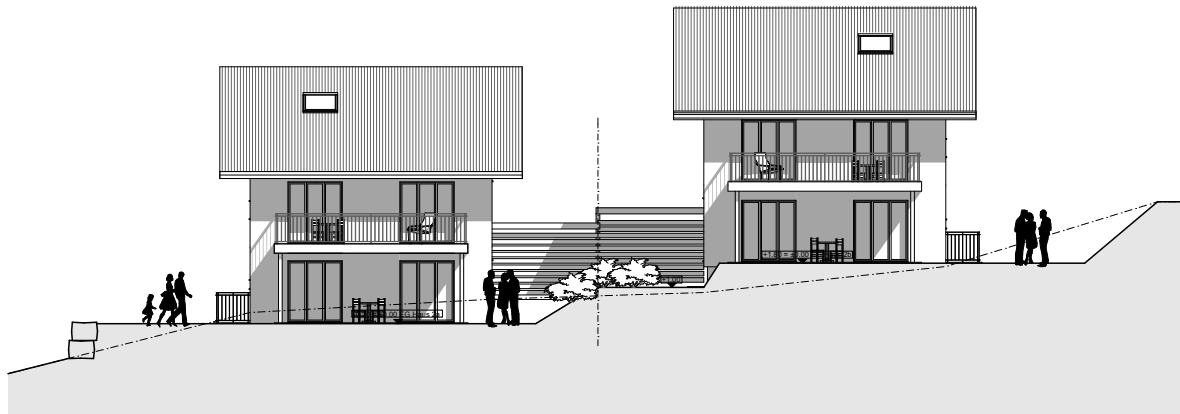
Süd-Fassade
