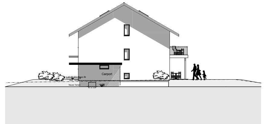
West-Fassade
